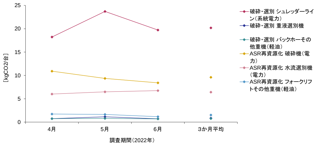
図 2-10 ELV の解体・破碎・ASR 再資源化による CO 2 排出量の推計結果の推移 (B 社)
